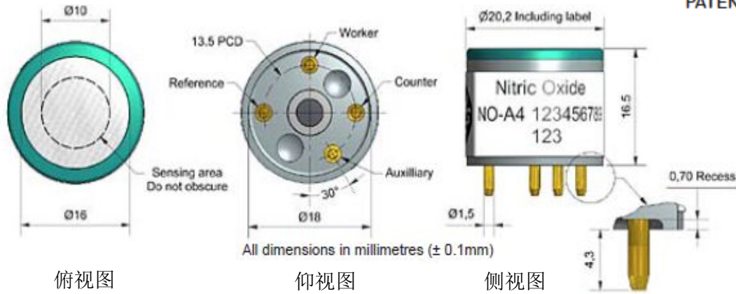
图1 NO-A4示意图
