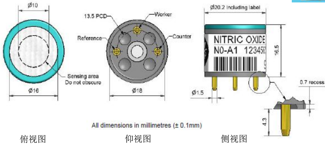
图1 NO-A1示意图
