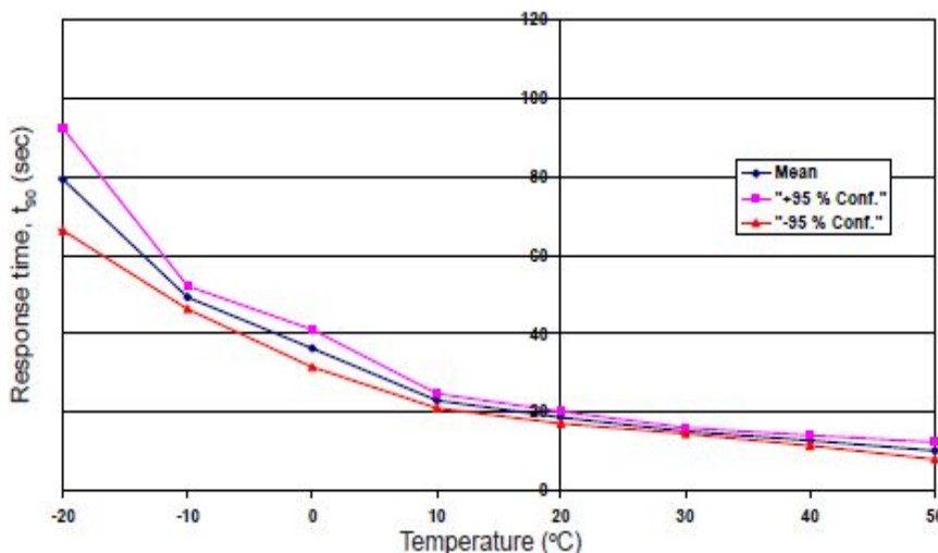
图4 响应时间 (t90) 温度特性
