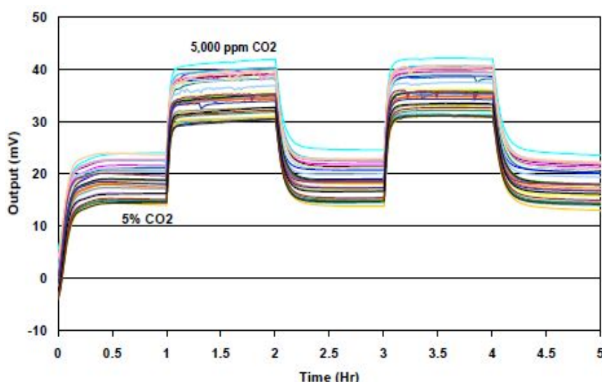
图3 迟滞
