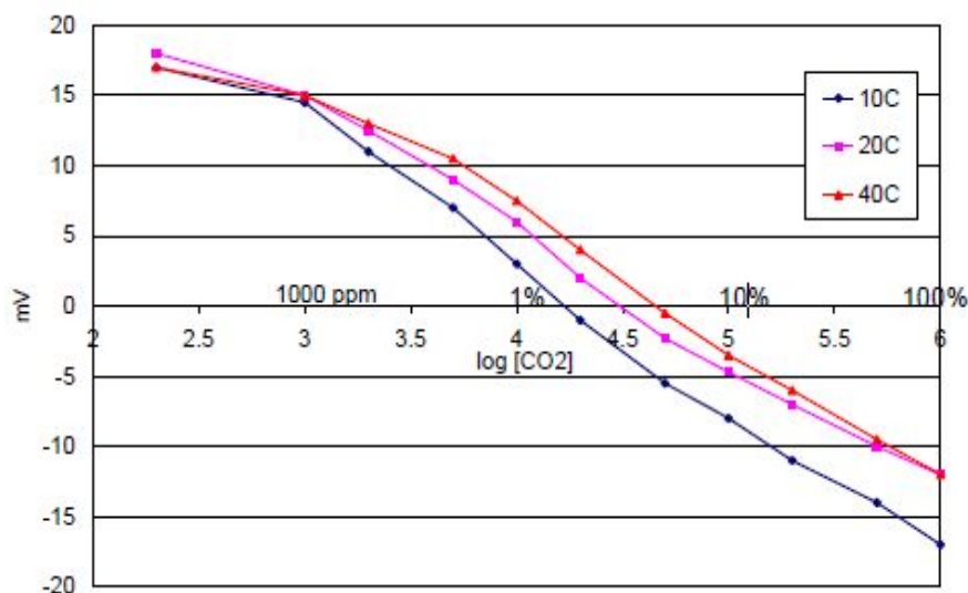
图2 主曲线
