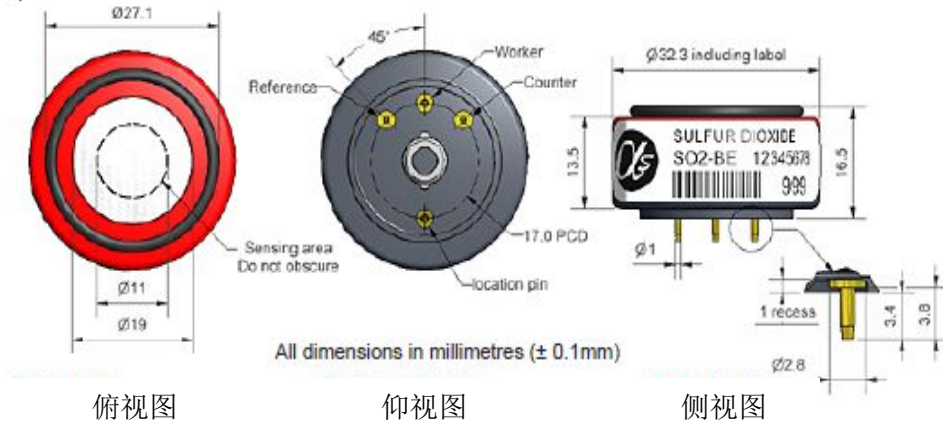
图1 SO2-BE示意图
