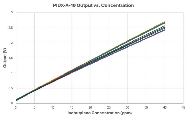
Fig. 1 PIDX-A-040 线性度(0-40 ppm)
