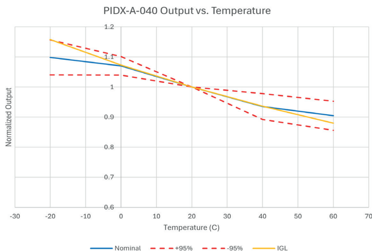
Fig. 2 灵敏度温度特性
