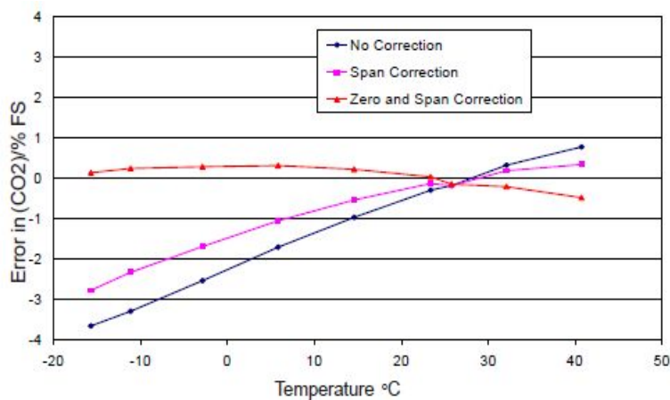
图4 温度补偿
