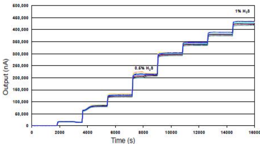
图4 高浓度反应
